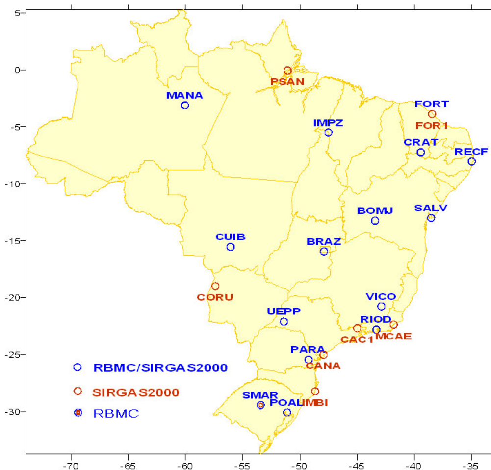
Figura 4 – Estações SIRGAS2000/RBMC.
