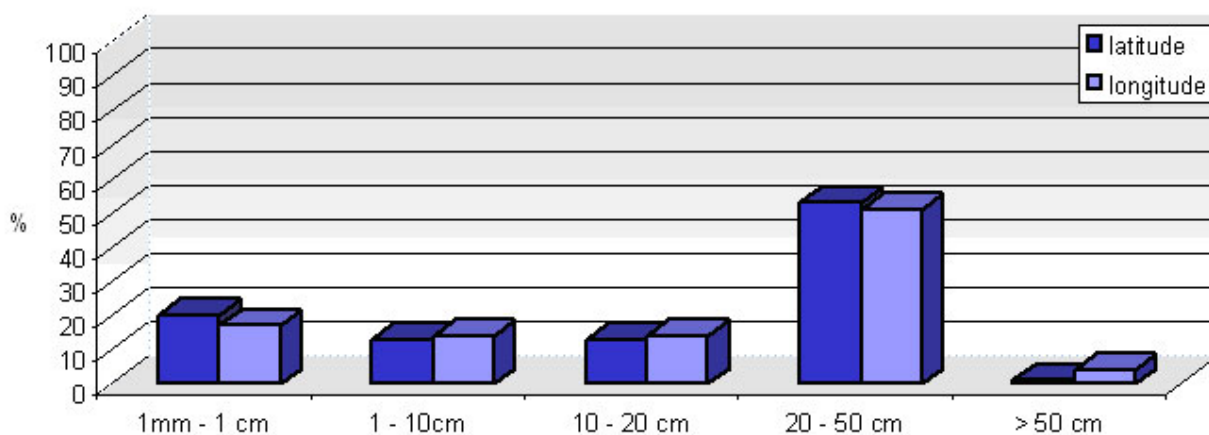
Gráfico 2 – Distribuição estatística dos desvios padrão das coordenadas de toda a rede.
