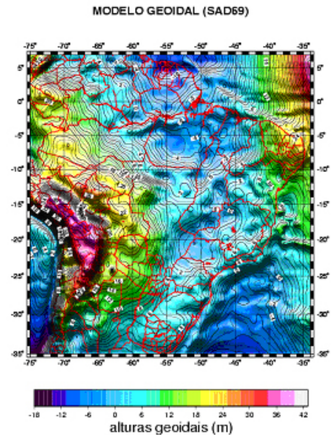
Figura 4 – Ondulação Geoidal – SAD69
