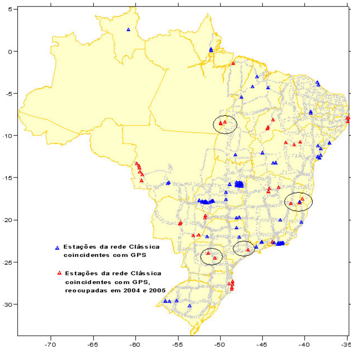
Figura 1 – Conexões entre as Redes Clássica e GPS.
